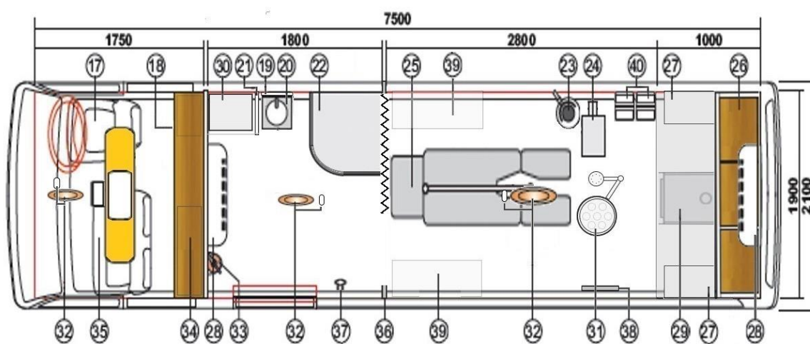
TAMPAK ATAS
