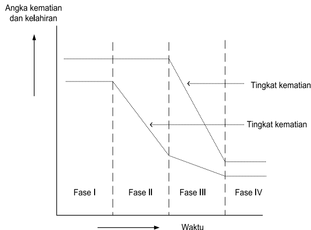
Gambar 2.10. Transisi Demografi
