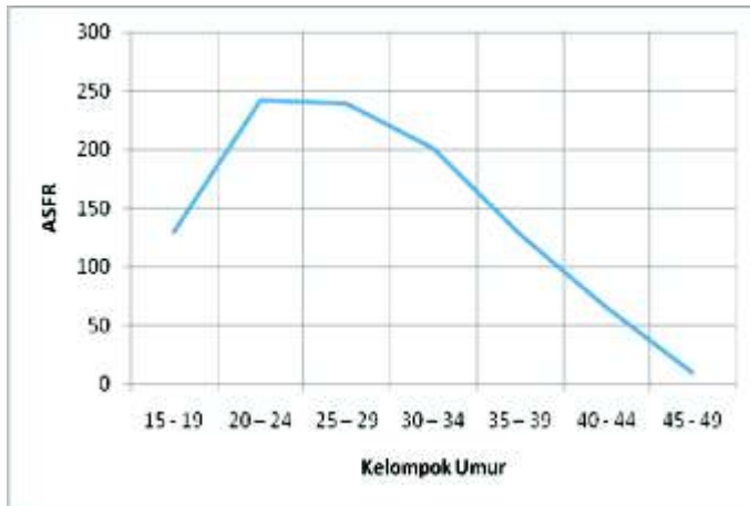
Gambar 2.2. Grafik ASFR
